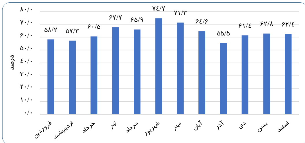
نمودار (۵-۱) میانگین روزانه رطوبت شهر بندرعباس در سال ۱۴۰۲
