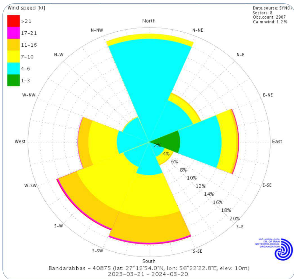
نمودار (۱-۶) گلباد سالانه شهر بندرعباس در سال ۱۴۰۲ (برحسب knot)
