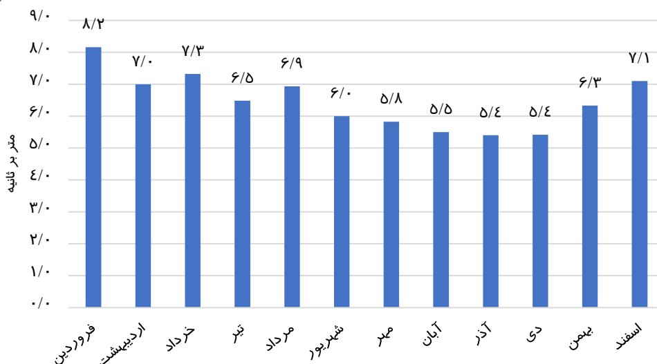
نمودار (۷-۱) میانگین روزانه سرعت باد بیشینه شهر بندرعباس در سال ۱۴۰۲
