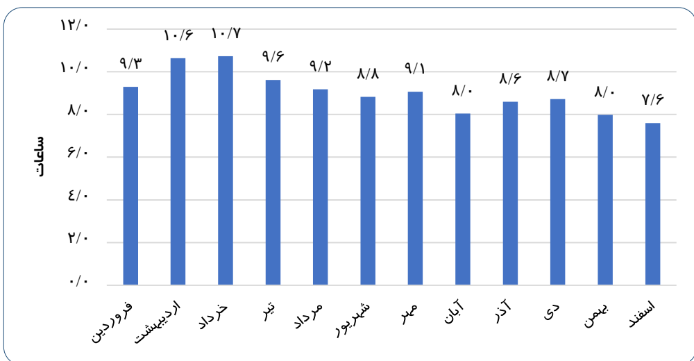
نمودار (۴-۱) میانگین روزانه ساعات آفتابی شهر بندرعباس در سال ۱۴۰۲
