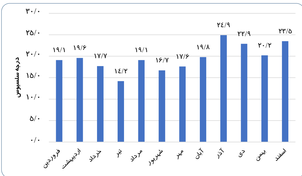
نمودار (۱-۳) دامنه دمایی ماهانه (اختلاف حداکثر و حداقل دمای مطلق) هوای شهر بندرعباس در سال ۱۴۰۲
