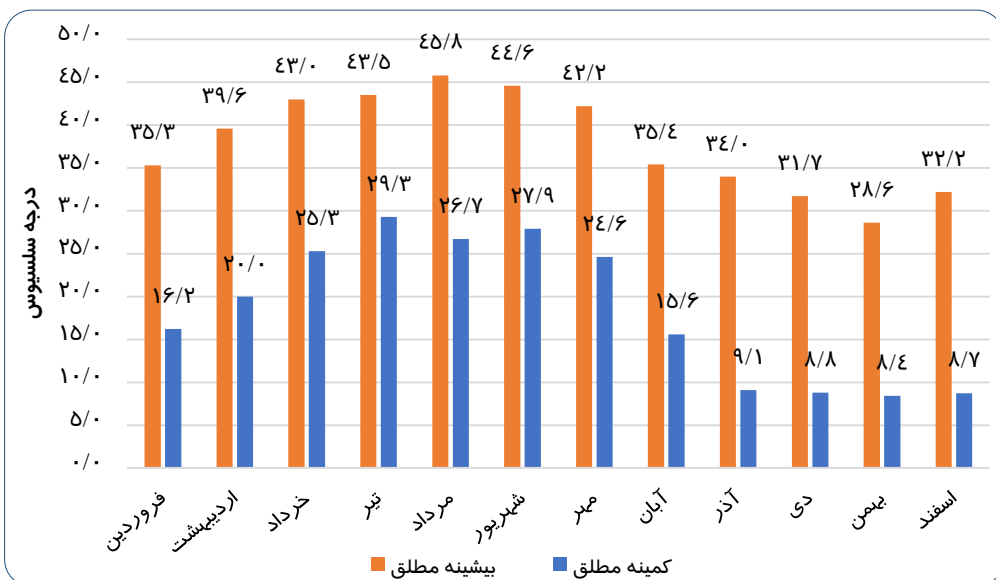
نمودار (۱-۲) کمینه و بیشینه مطلق دمای ماهانه شهر بندرعباس در سال ۱۴۰۲
